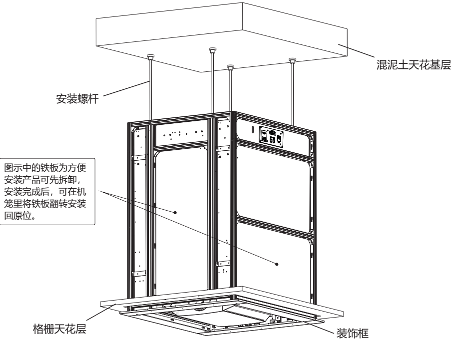
(安装示意图)
